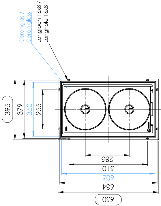
Draufsicht / Top view Variante B / Version B
