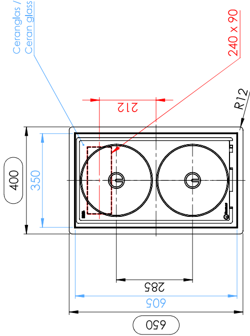
Draufsicht / Top view Variante A / Version A
